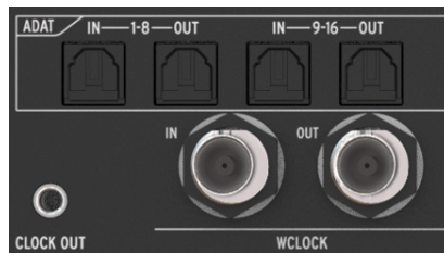
ADAT und Word Clock-Ports auf der Rückseite
