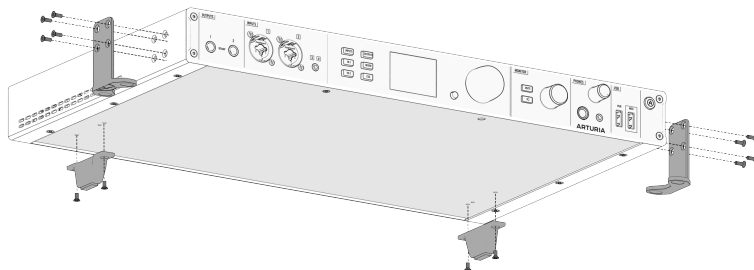
L'AudioFuse 16Rig configurée pour une utilisation sur table
