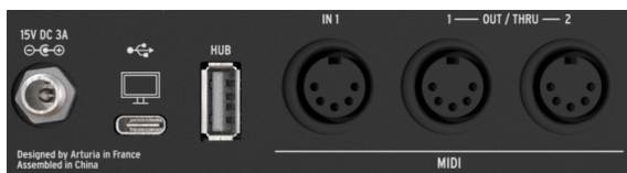
リアパネルの MIDI、USB、電源コネクタ
