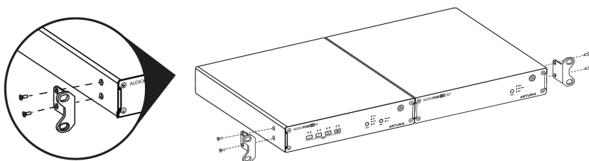
L'AudioFuse X8 IN configurée pour une utilisation en rack
