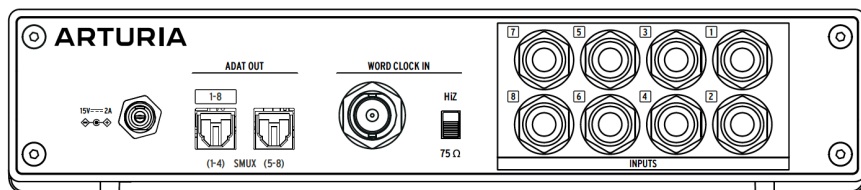
Le panneau arrière de l'AudioFuse X8 IN
