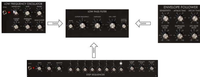
Filter MINI signal flow
